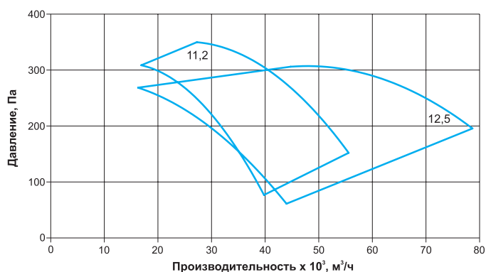
Сводная аэродинамическая характеристика вентиляторов POCA-SMF № 11,2-12,5 (1000 об/мин)
